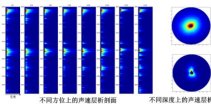
不同方位上的声速层析剖面
