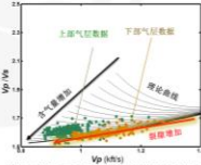
模拟含气页岩的纵、横波测井数据
